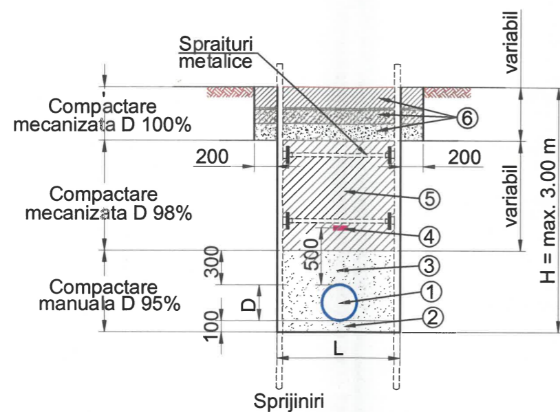
DETALIU SAPATURA TIP 1 - Pozare conducta alimentare cu apa in transee cu H max = 3,00 m
